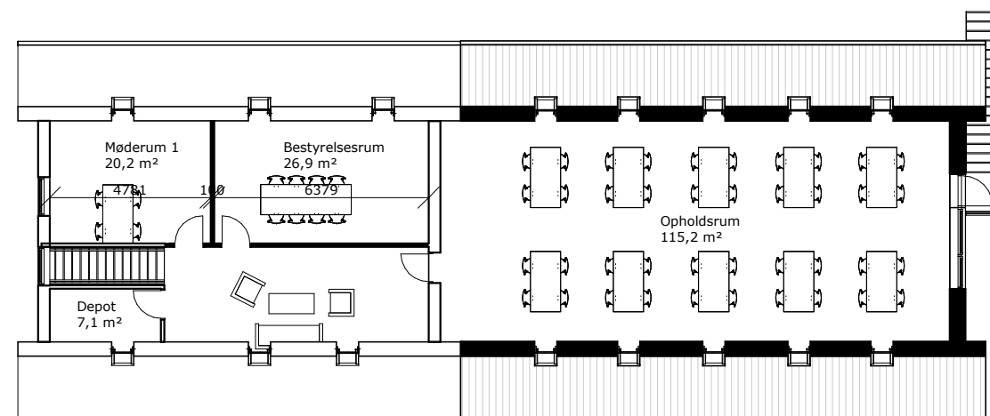
Ny 1. Sal
