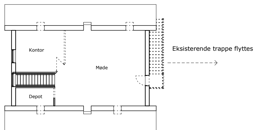
Nedbrydningsplan 1. Sal
